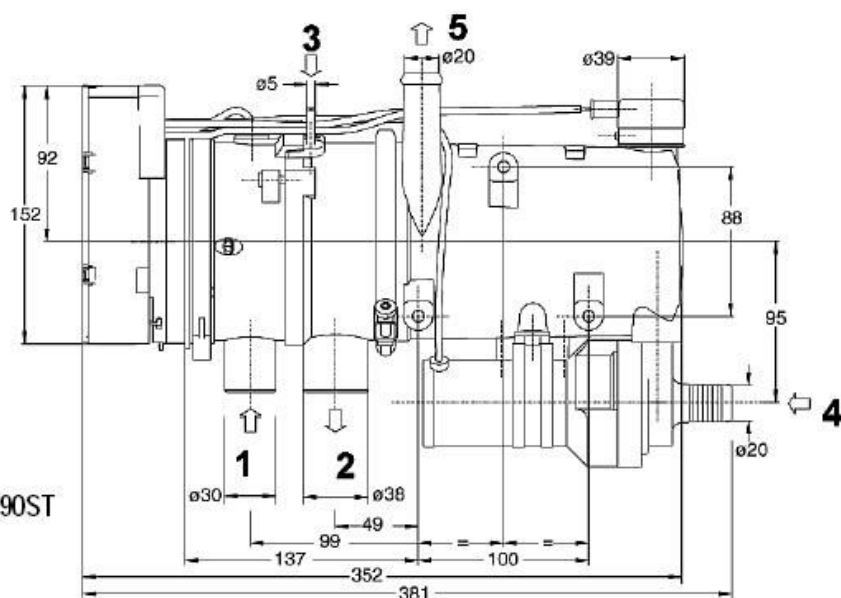
Рис. 2 Габариты подогревателя
